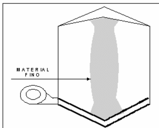
Figura b: Ubicación del material fino en un silo.
