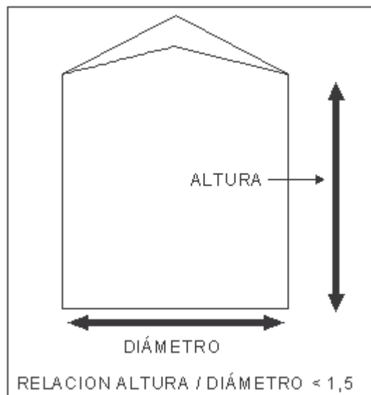
Figura a: Relación altura diámetro de un silo
